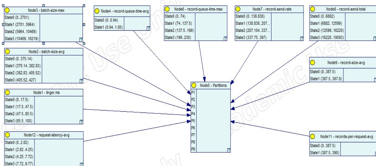
Рисунок 4 – Структура мережі Байєса для підтримки прийняття рішення щодо оптимальної кількості розділів Apache Kafka-продюсера
