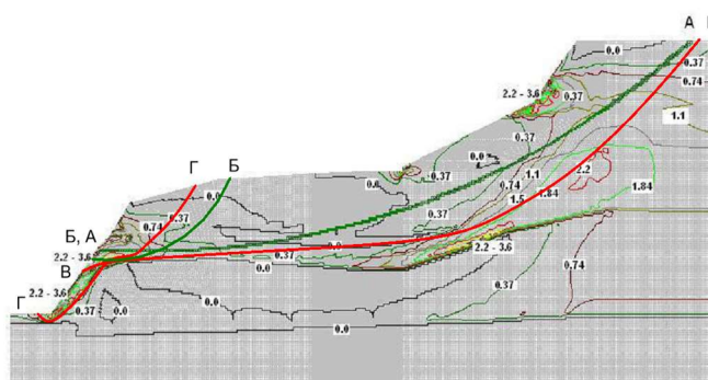
Рисунок 6 – Розрахунковий профіль I-I, поверхні зсуву А-А, Б-Б, В-В, Г-Г, ізолінії інтенсивності пластичних деформацій, %
