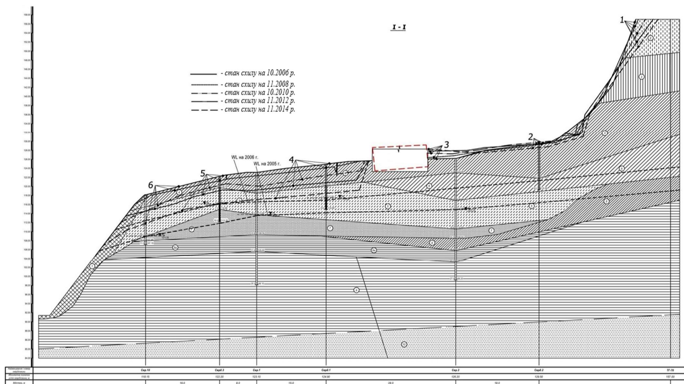
Рисунок 5 – Інженерно-геологічний розріз I-I
