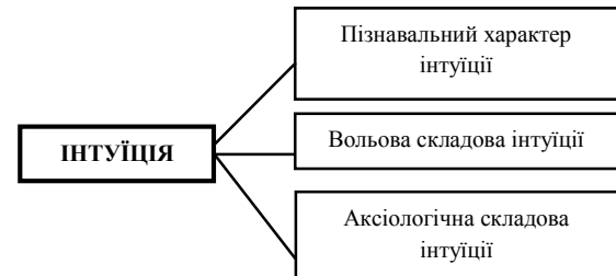
Рис.1. Складові інтуїції
