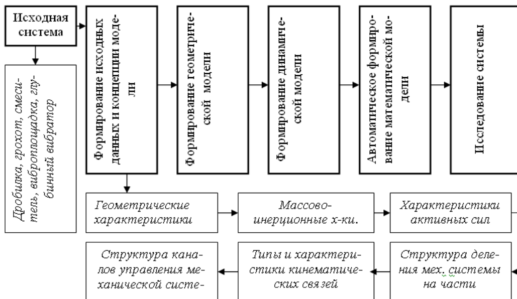
Рис. 2. Технология моделирования механического оборудования в программном комплексе EULER
