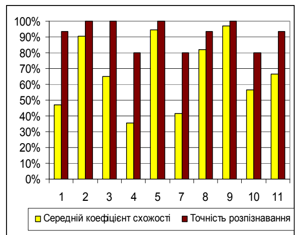
Рис. 1. Гістограма загальної точності розпізнавання та середнього коефіцієнта схожості зображень Yale Faces Data Base
